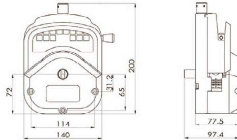
YZ35-Aluminum Alloy
