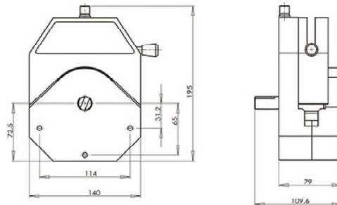
YZ35-Aluminum Alloy
